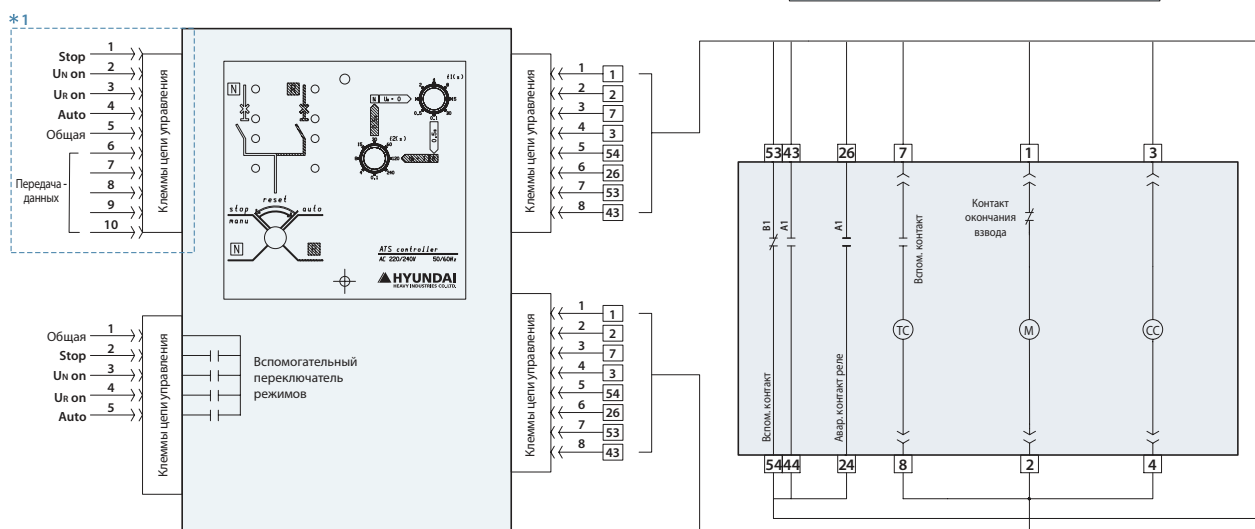
Схема подключения доп. компонентов к АВР
