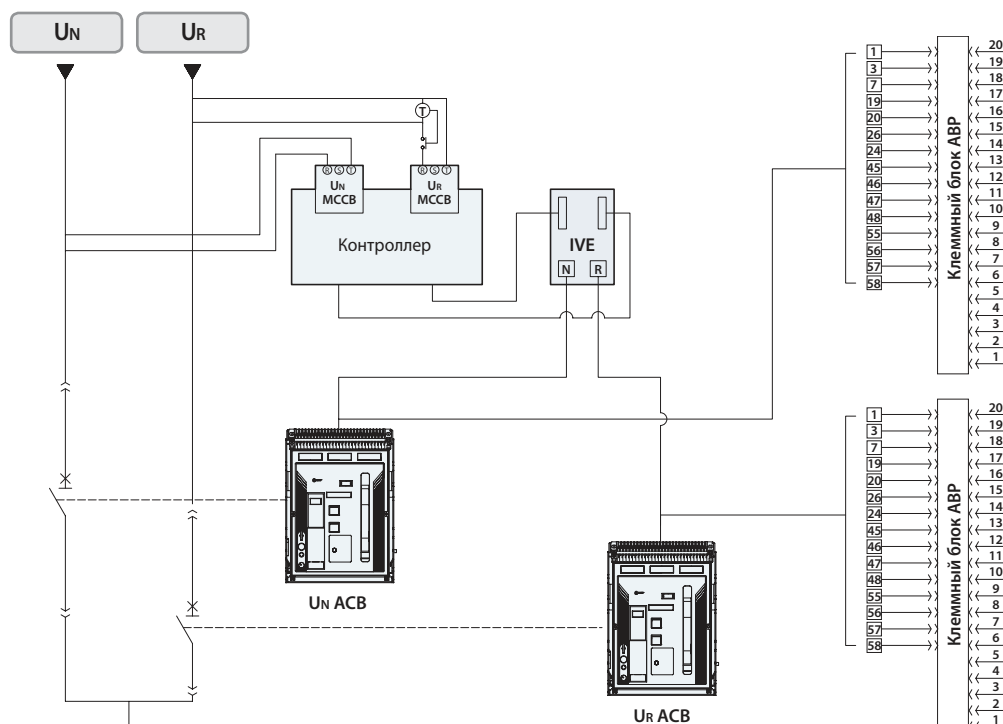
Схема подключения АВР с двумя выключателями
